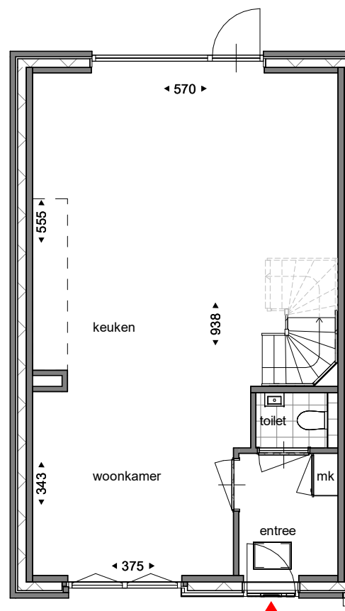
begane grond
