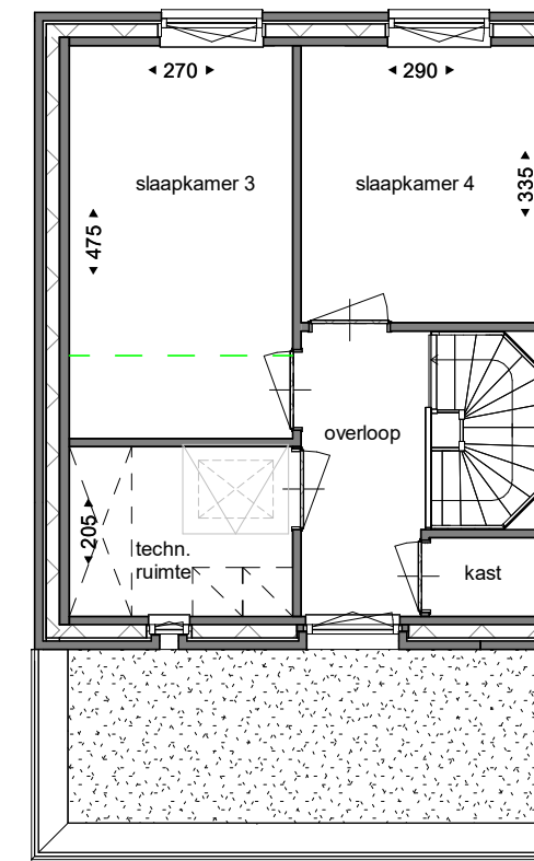
tweede verdieping
